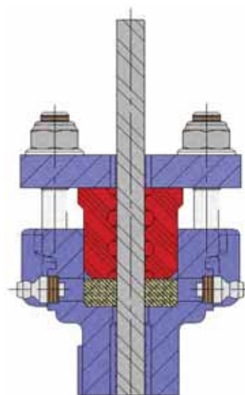
Секция F-F
