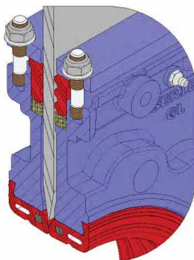
Деталь G
