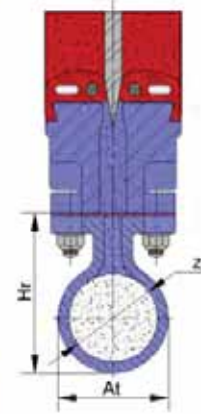
Секция B-B
